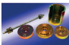
Ściągacz tulei tylnej belki (środkowa) BMW 5 (E 60, E61) BMW 6 (E63, E64) Symbol: WAR 520 Cena: 184,81 zł
